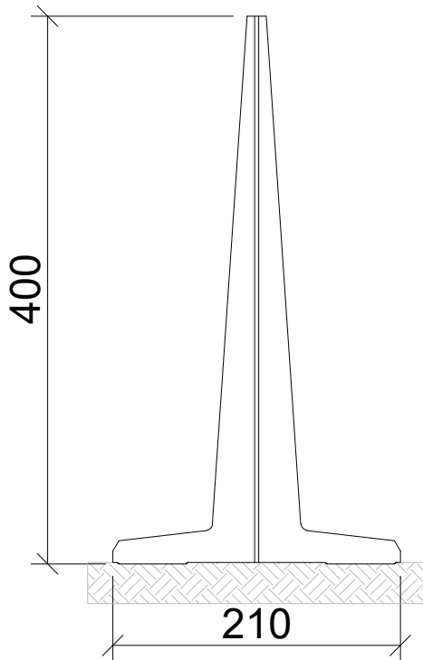
SEZIONE
